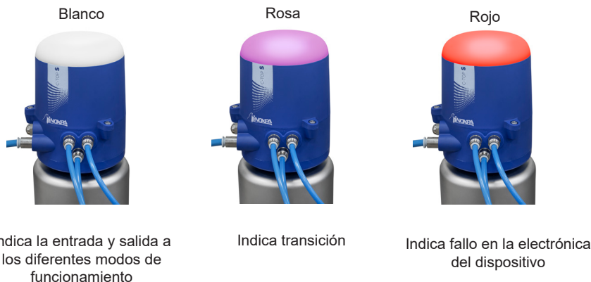
Módulo electrónico
